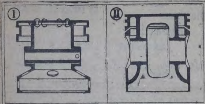
Fig. 4. — Dos modelos de pistones de aluminio de uso corriente
